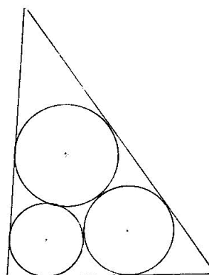
Problème de Malfatti
